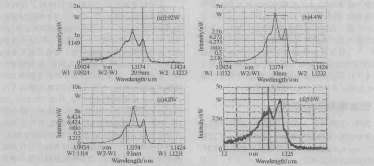
图 3 不同泵浦功率下测得的第一级 Stokes 光谱 Fig.3 The first-order stokes spectra with different pump power
