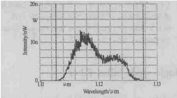
图 4 新的实验条件下的 Stokes 光谱图 Fig. 4 Stokes spectrum at different experiment condition
