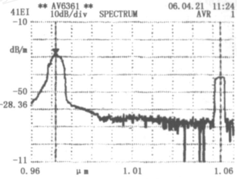
图 4 采用方案二时的激光光谱( I=1400\text{mA} )
