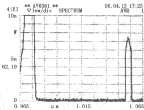
图 3 采用方案一时的激光光谱( I=1400\text{mA} )
