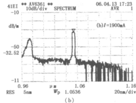
图 5 采用方案三时的激光光谱
