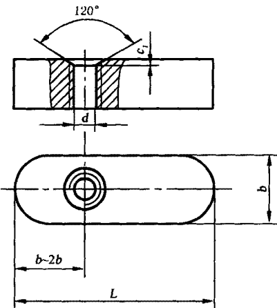
图 A.1 起键螺孔的位置
